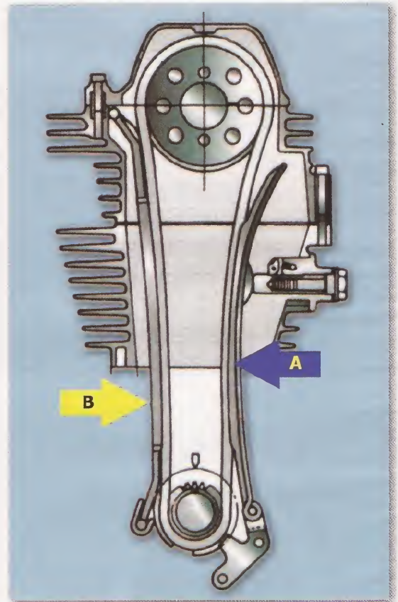
A. Tensor B. Guía de cadenilla
